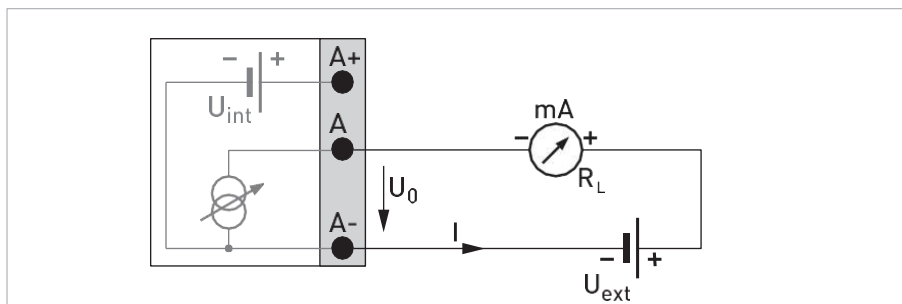
A Figura 4-14: saída de corrente I passiva p
