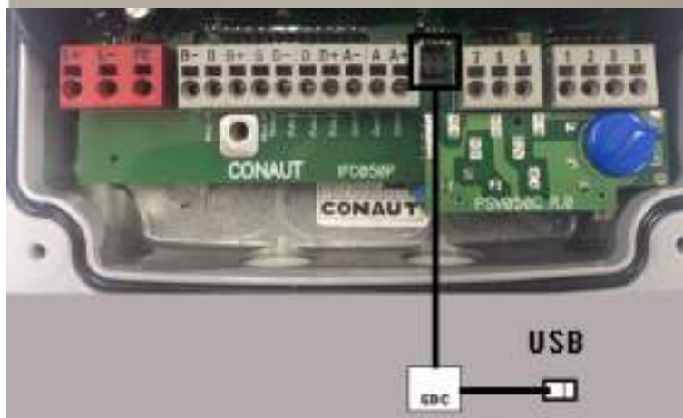
Conexão ao Terminal GDC do IFC050P
