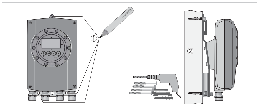
Figura 3-1: fixação da caixa
