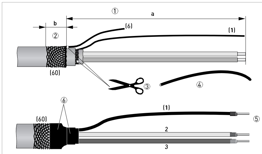
Figura 4-5: Preparação cabo de sinal A, ligação ao sensor de vazão
