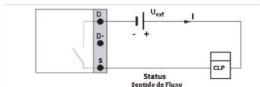
Figura 4-16: Sentido de Fluxo / saída passiva P_p
