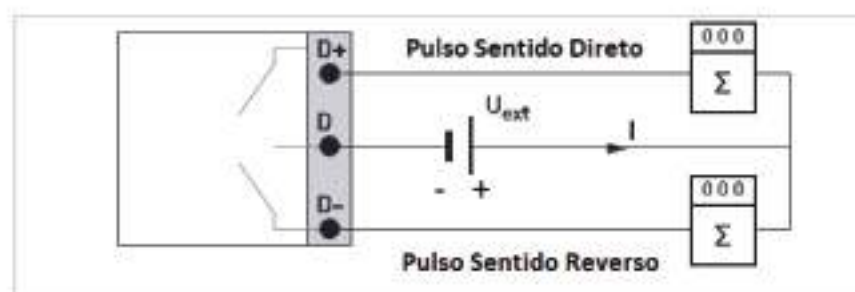
A Figura 4-15: Pulso / Frequência, saída passiva P_p
